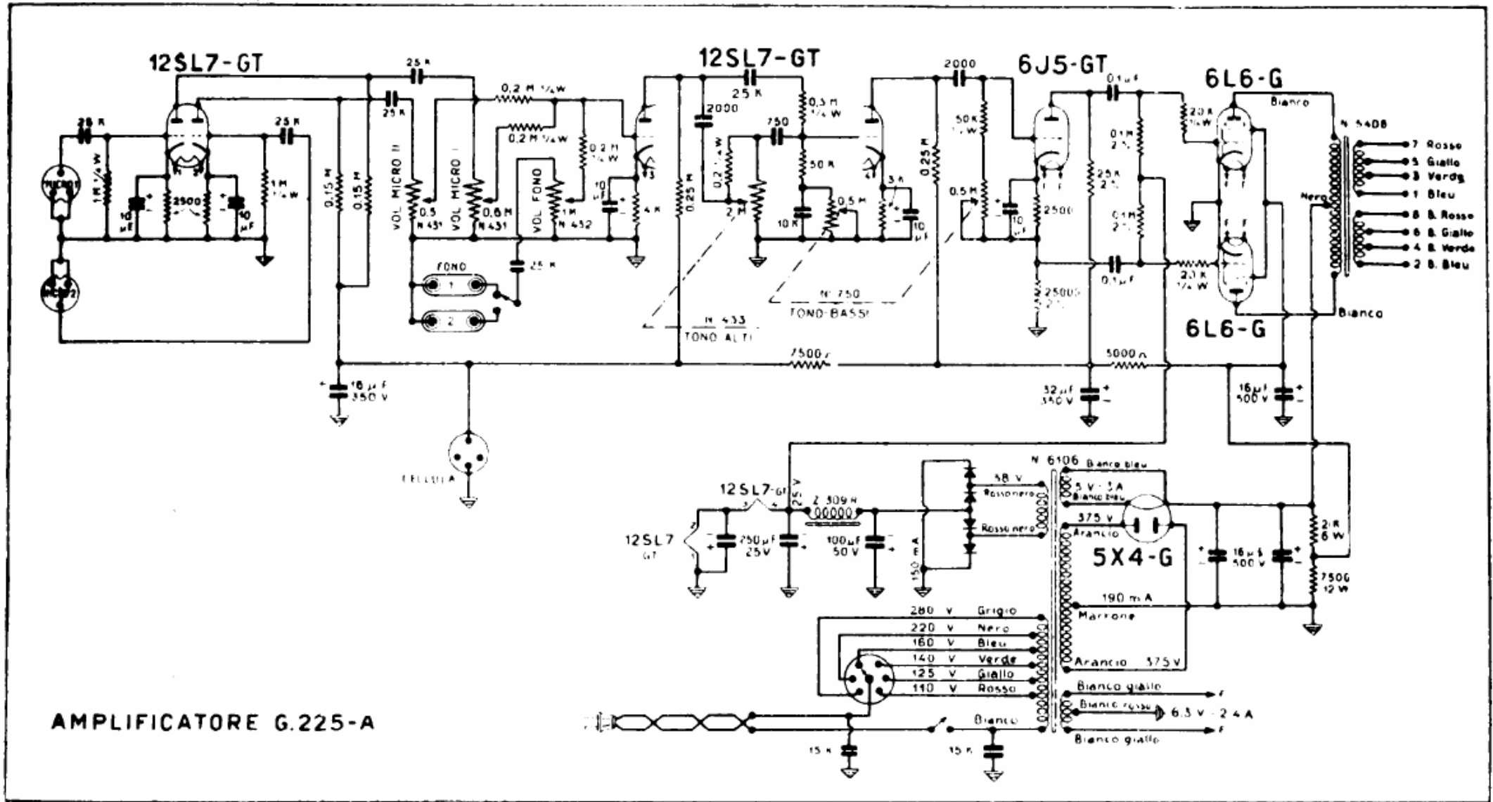
Lo schema elettrico
